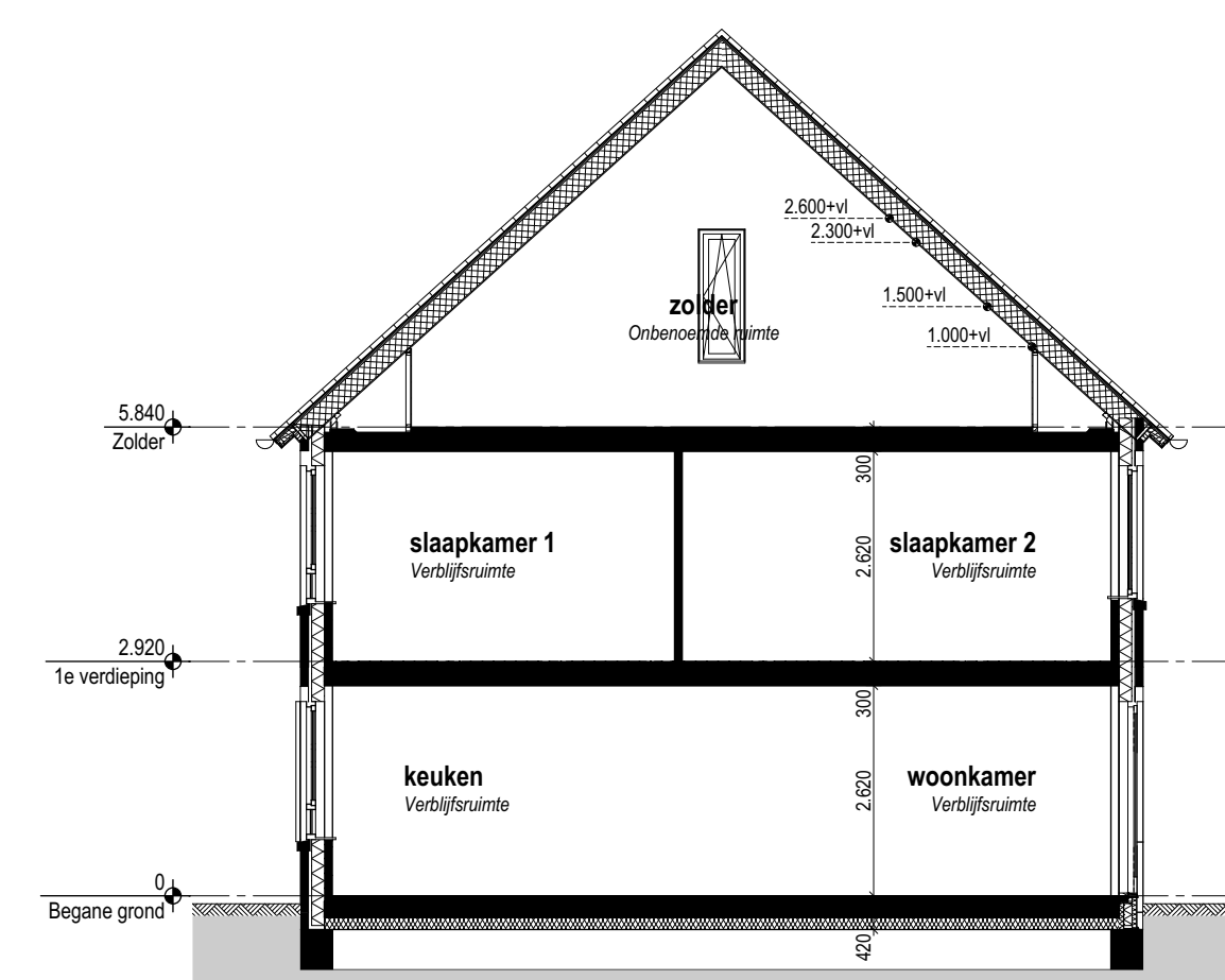
Doorsnede B-B (1:100)
