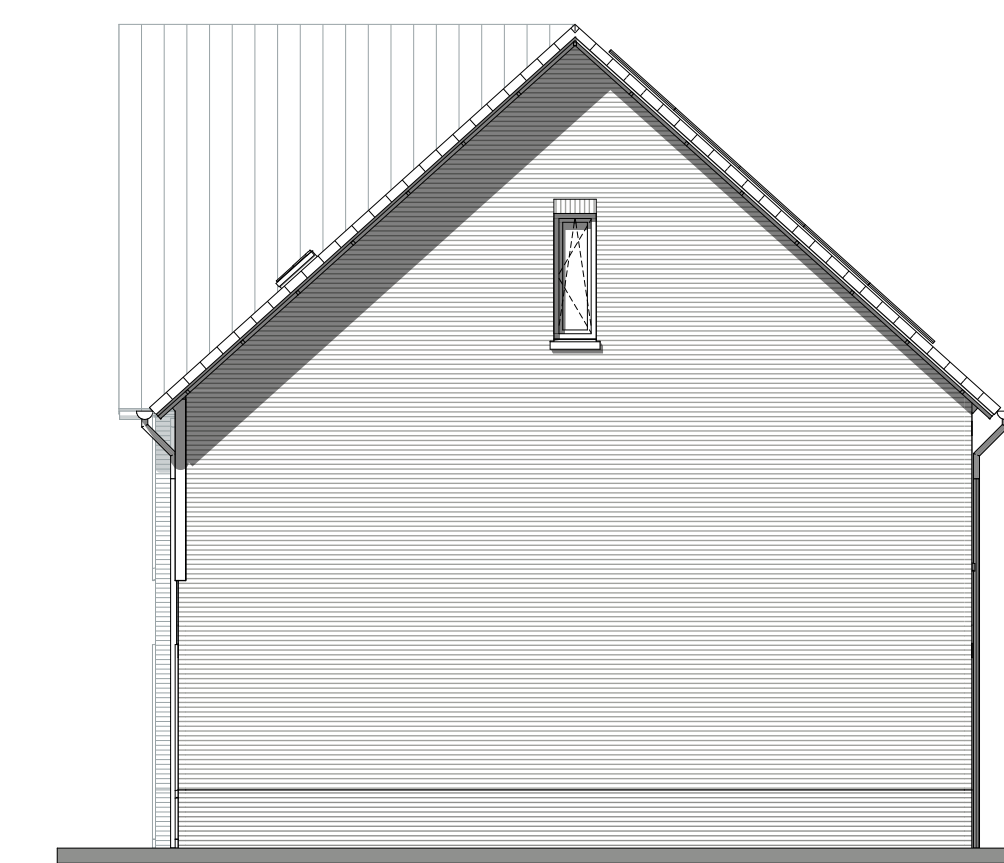
Rechter zijgevel (1:100)
