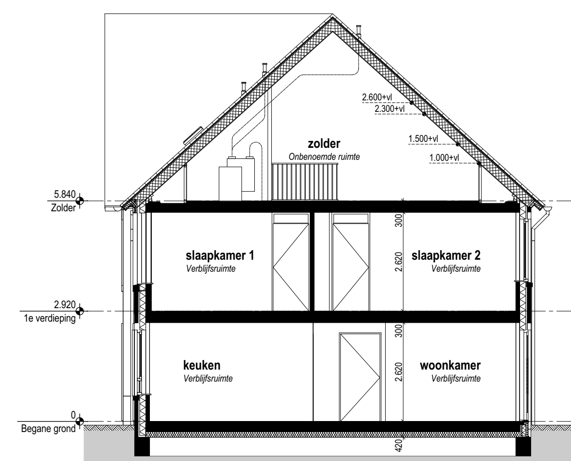
Doorsnede A-A (1:100)
