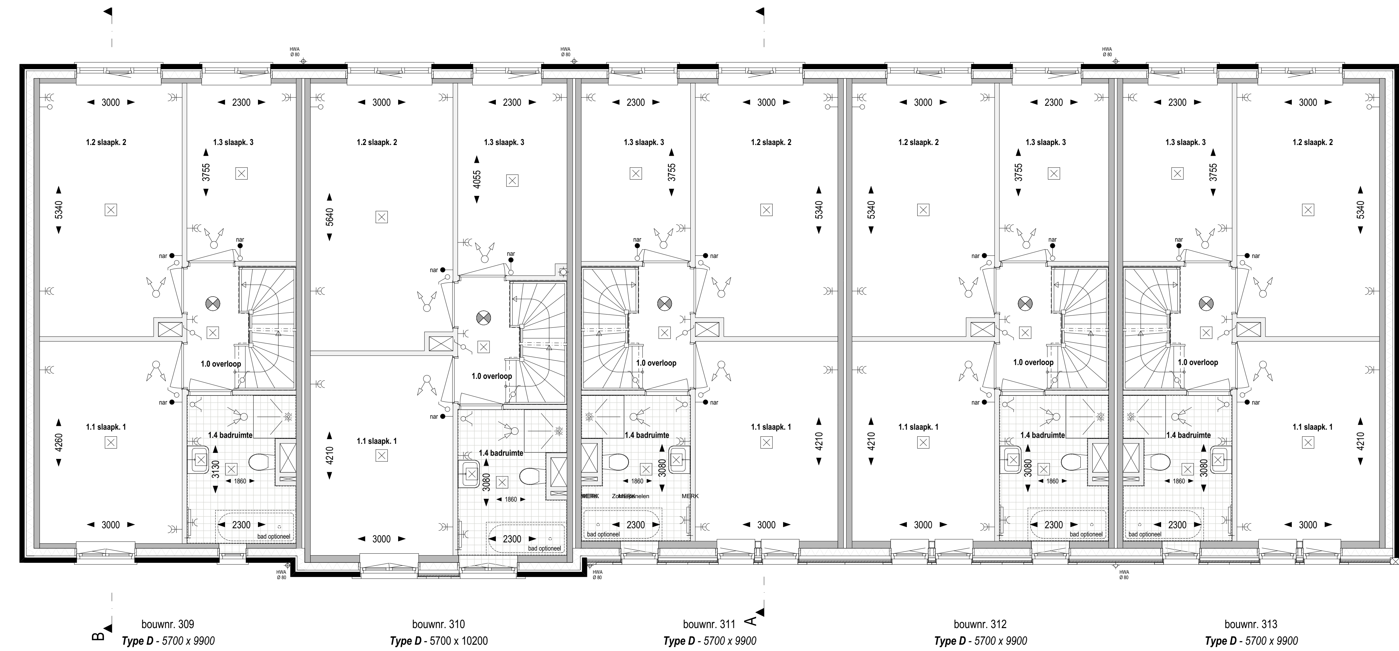
1e Verdieping +2.920 (1:50)
